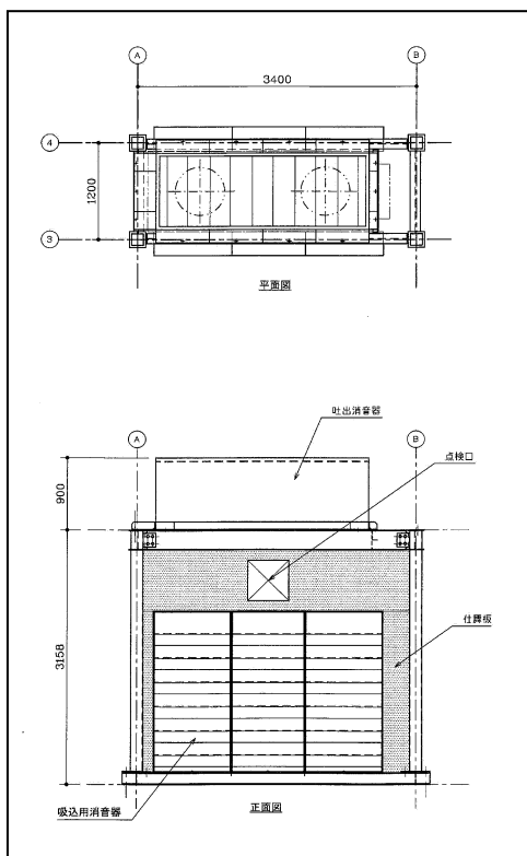
参考図 (防音性能15dB(A)タイプ)
