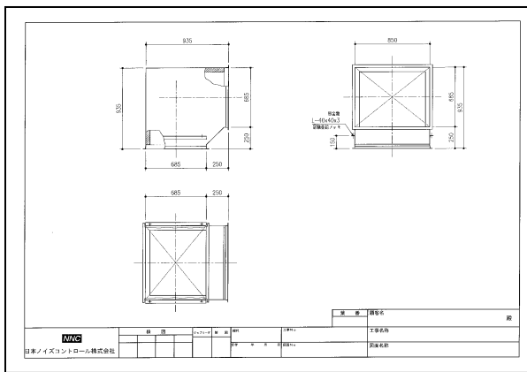
しずかE型 標準寸法図
