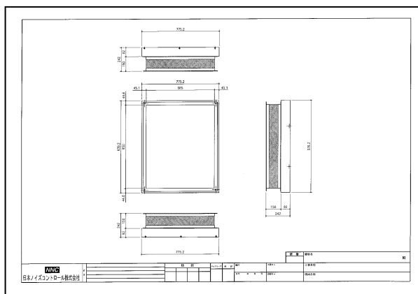
接続フランジ寸法図 (オプション)
