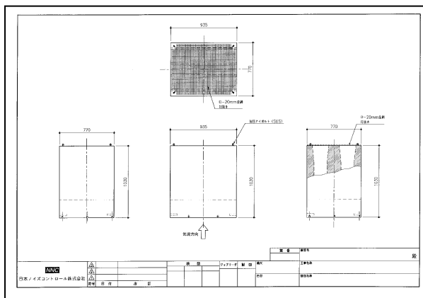
“しずか”S型 標準寸法図
