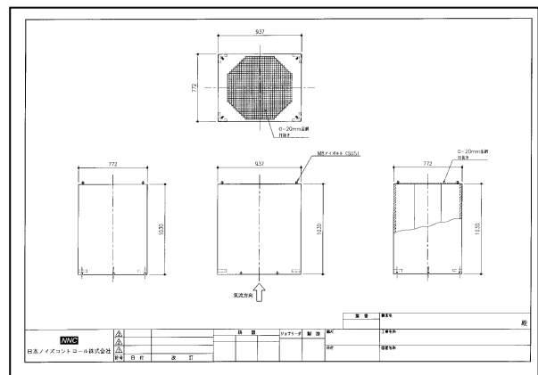
“しずか”SII型 標準寸法図
